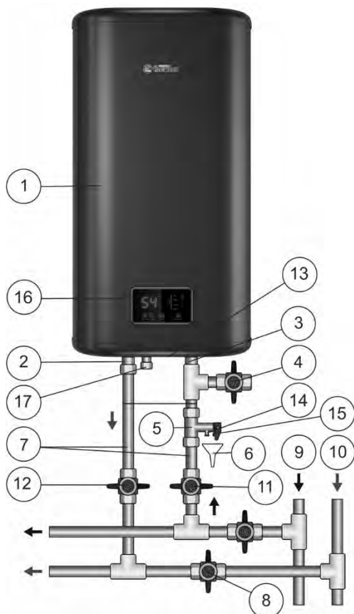
Bild 1. Wasseranschluss
